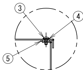
カブセ蓋取付け部詳細図
